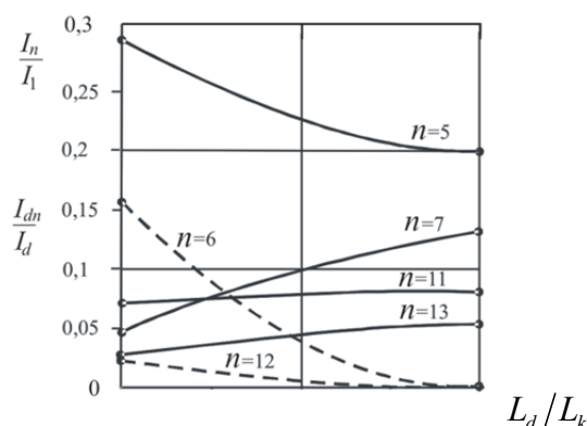
Рис. 3. Зависимость гармоник сетевого тока и тока нагрузки от отношения L_d/L_k
