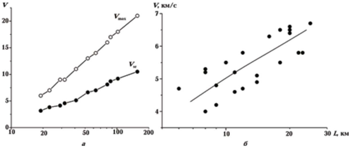
Рис. 7. Зависимости средней V_{sr} и максимальной V_{max} скоростей разрыва от длины разрыва L : a — модель; b — результаты анализа таблиц из работы [Горбунова и др., 1992].
