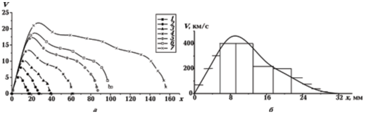
Рис. 4. Зависимости скорости перемещения края разлома от расстояния по разлому: a — компьютерный расчет ("скорости" и расстояния даны в клеточно-автоматных единицах); b — физический эксперимент [Виноградов, 1976] (1—7 — то же, что и на рис. 3).
