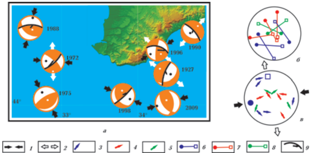
Рис. 6. Поля напряжений, определенные по механизмам очагов землетрясений: а — эпицентры и механизмы очагов; б — стереодиаграмма осей сжатия (кружок) и растяжения (квадрат) в очагах; в — стереодиаграмма векторов и осей главных нормальных напряжений для совокупности механизмов очагов; 1, 2 — проекции осей главных нормальных напряжений на горизонтальную плоскость (1 — сжатия; 2 — растяжения); 3—5 — векторы подвижек с преобладанием определенной компоненты смещения (3 — сдвиговой; 4 — взбросовой; 5 — сбросовой); 6—8 — оси сжатия и растяжения для полей (6 — сдвигового типа; 7 — взбросового типа; 8 — сбросового типа); 9 — плоскость сейсмогенного разрыва.
