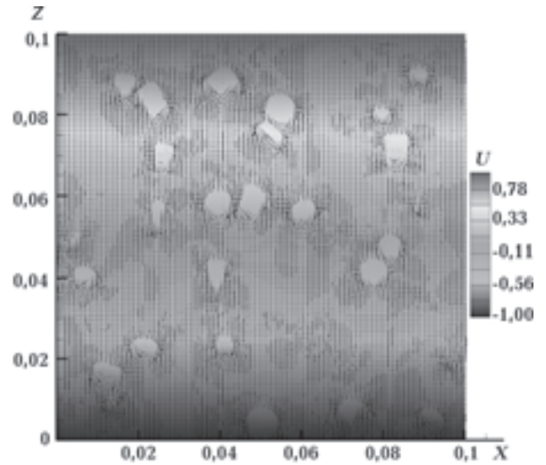
Рис. 4. Распределение потенциала и вектора плотности электрического тока.
