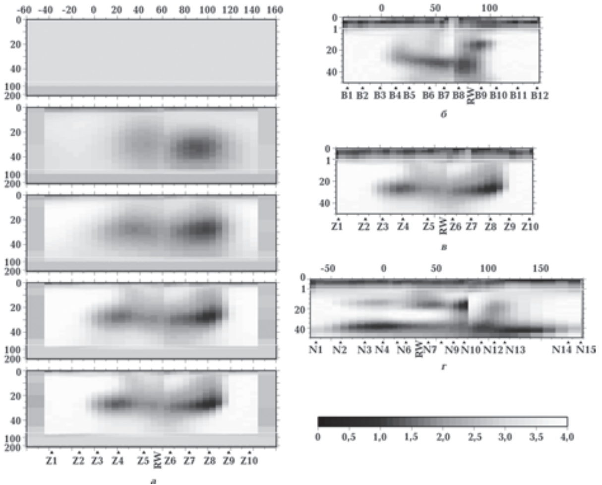
Рис. 3. Результаты 2D+ инверсии 8-компонентного ансамбля МТ/МВ данных на северных профилях эксперимента KIROVOGRAD: a — разрезы сопротивления, Ом·м (lg-шкала, в нижней части модели другой вертикальный масштаб) на профиле ЖИЗДРА для различных итераций решения обратной задачи (сверху вниз 0, 22, 38, 58 и 68); б — г — итоговые разрезы электрического сопротивления, Ом·м (lg-шкала, в верхней части модели мощностью 1 км другой вертикальный масштаб) для профилей КИРОВ ( б ), ЖИЗДРА ( в ) и НАВЛЯ ( г ); начало горизонтальных координат, км — на меридиане 34° в.д.; RW указывает на положение ж/д Москва—Киев.
