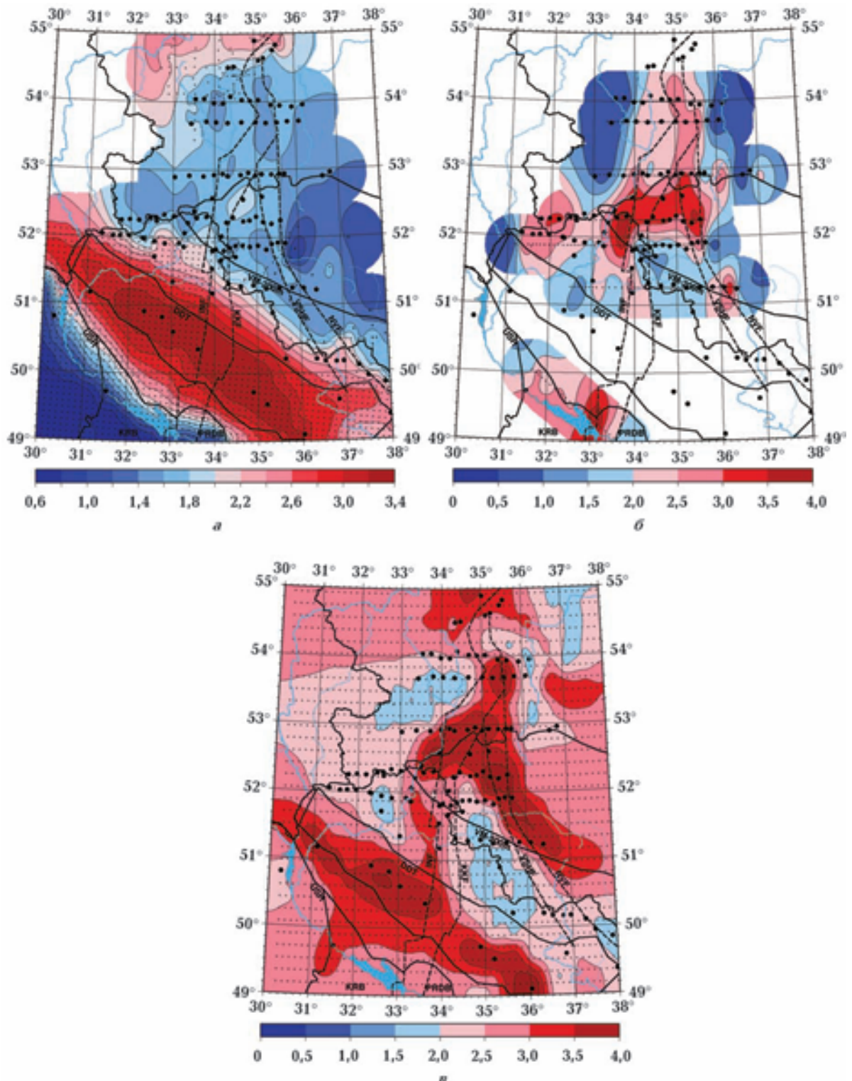
Рис. 4. Карты суммарной продольной проводимости (lg-шкала) на западном склоне ВМ и сопредельных территориях. См: а — осадочный чехол по эффективным оценкам в точках синхронных зондирований KIROVOGRAD (черные кружки) и результатам комплексного анализа ранее полученных электроразведочных данных (крестики); б — земная кора в диапазоне глубин 15—50 км по результатам 2D+ инверсии 8-компонентных ансамблей МТ/МВ данных (крестики — точки оценивания на профилях зондирований KIROVOGRAD); в — земная кора в пленочной аппроксимации (глубина пленки — 20 км) по результатам квази-3D инверсии данных горизонтального МВ отклика для синхронных зондирований KIROVOGRAD (крестики — центры ячеек инверсии). Легенда тектонических границ (черные линии) дана на рис. 1.
