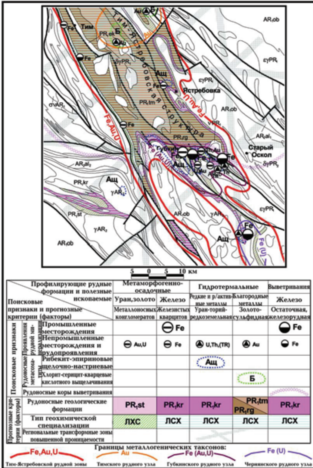
Рис. 3. Оскольский рудный район КМА. Карта закономерностей размещения полезных ископаемых докембрийского фундамента.
