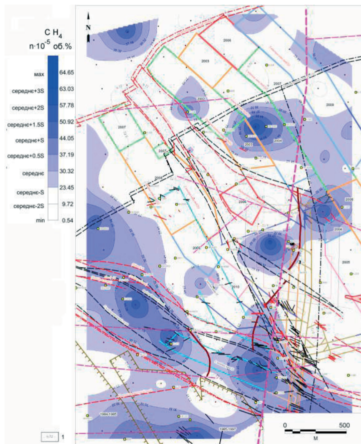
Рис. 13. Схема пространственного распределения показателей содержания метана в подгрунтовом воздухе на участке шахты «Краснолиманская»: 1 – изолинии показателей содержания метана \text{CH}_4 \cdot (n \cdot 10^{-5} \text{ об. } \%)
