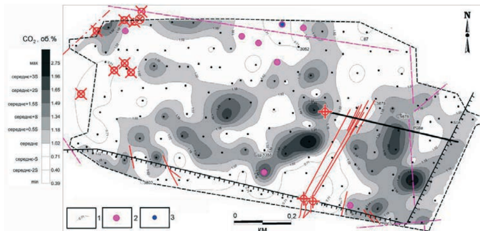
Рис. 10. Схема пространственного распределения показателей содержания углекислого газа, водорода и гелия в подгрунтовом воздухе на Северном детализационном участке шахты им. Засядько: 1 – изолинии показателей содержания углекислого газа (CO 2 ); пункты наблюдений, где концентрация атмогеохимического показателя превосходит чувствительность прибора: 2 – водород (H 2 ), 3 – гелий (He)
