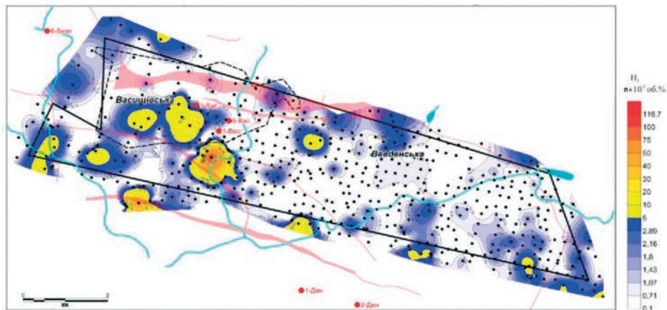
Рис. 7. Схема распределения показателей содержания водорода в подгрунтовом воздухе на Васищевской площади
