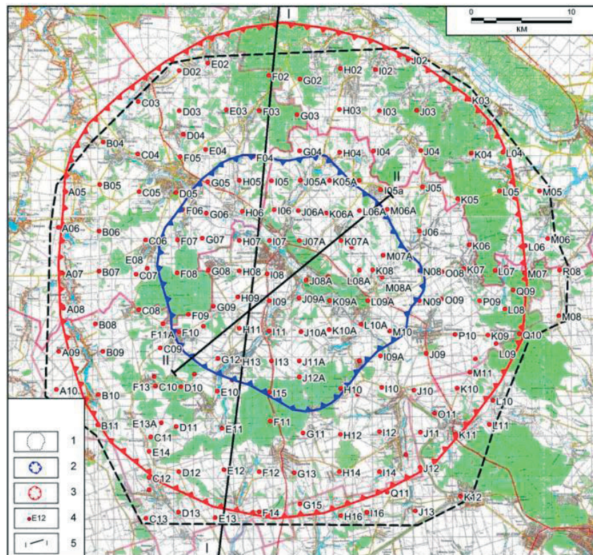
Рис. 1. Карта пространственного размещения пунктов наблюдений СТАГГИ на Болтышской импактной структуре (на топографической основе м-ба 1 : 100 000): 1 – границы площади исследований; контуры: 2 – кратера, 3 – предполагаемого цокольного вала; 4 – пункты наблюдений и их номера; 5 – профиль и его номер
