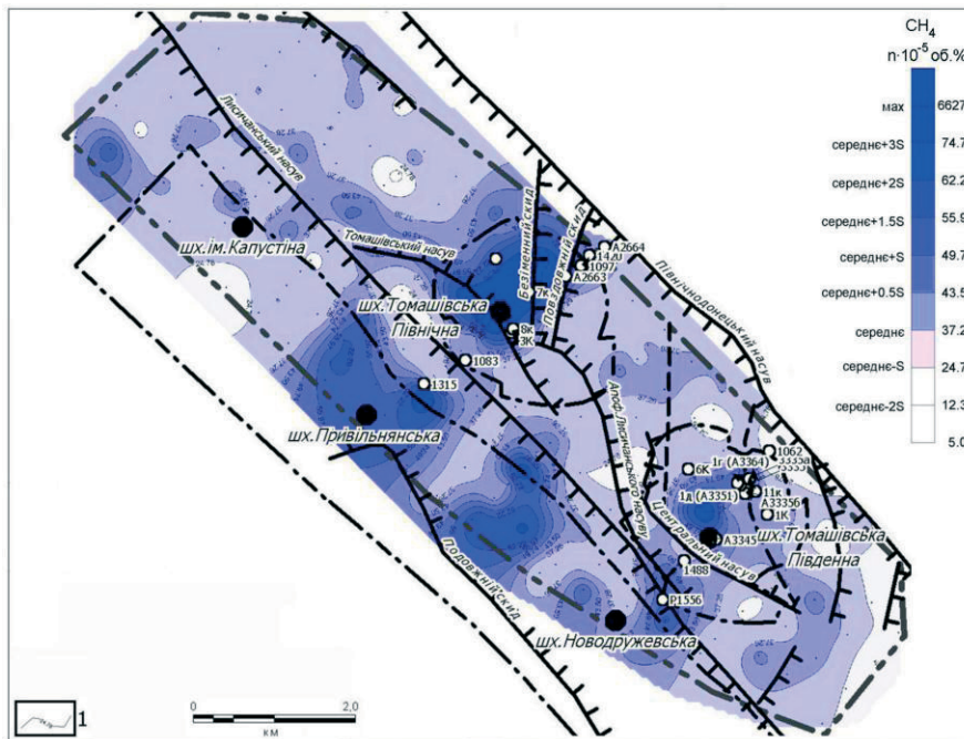
Рис. 9. Схема пространственного распределения показателей содержания метана в подгрунтовом воздухе на Томашевской площади: 1 – изолинии показателей содержания метана CH_4 \cdot (n \cdot 10^{-5} об. %)
