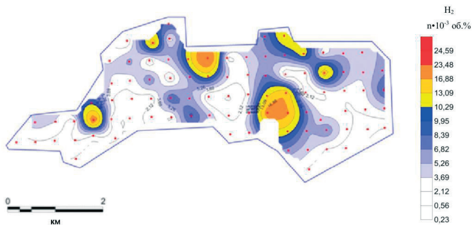
Рис. 3. Схема пространственного распределения показателей содержания водорода в слое донных отложений на структурах Субботина, Морская, Абиха
