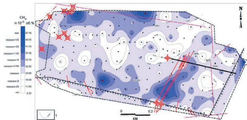
Рис. 11. Схема пространственного распределения показателей содержания метана в подгрунтовом воздухе на Северном детализационном участке шахты им. Засядько: 1 – изолинии показателей содержания метана CH 4 · (n · 10 -5 об. %)
