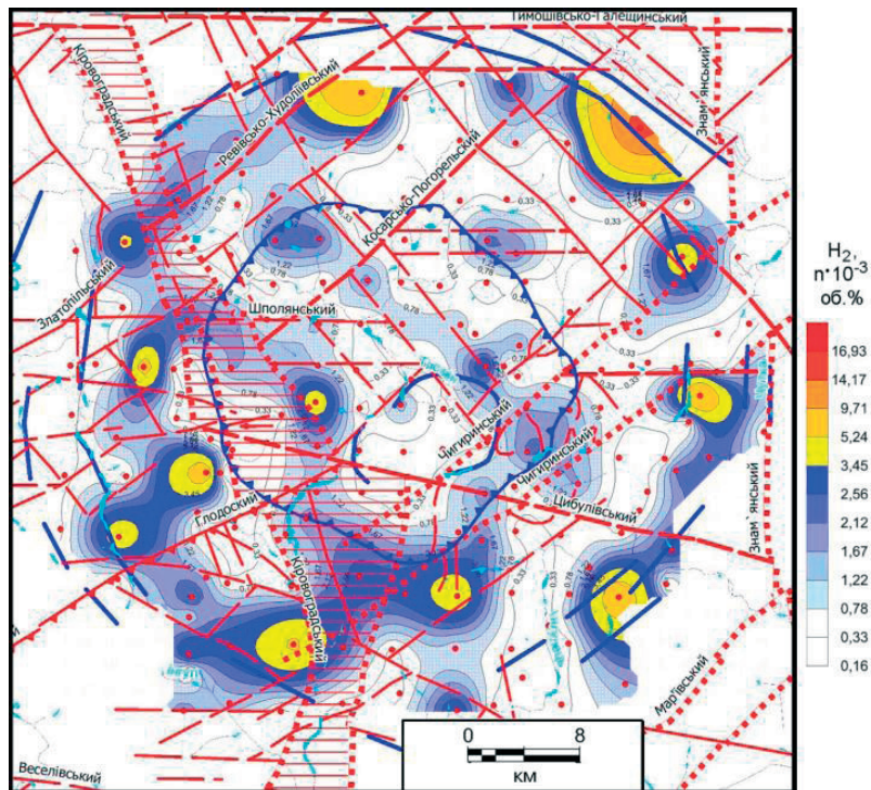
Рис. 2. Схема пространственного распределения показателей содержания водорода в подгрунтовом воздухе на Болтышской импактной структуре: 1 – пункты наблюдений СТАГГИ; 2 – контуры площади исследований; 3 – контуры Болтышской импактной структуры; разломы и их названия: 4 – взросы, 5 – сбросы, 6 – главные, 7 – второстепенные; 8 – зона Криворожского глубинного разлома; 9 – фрагменты кольцевых структур по результатам дешифрирования МКЗ
