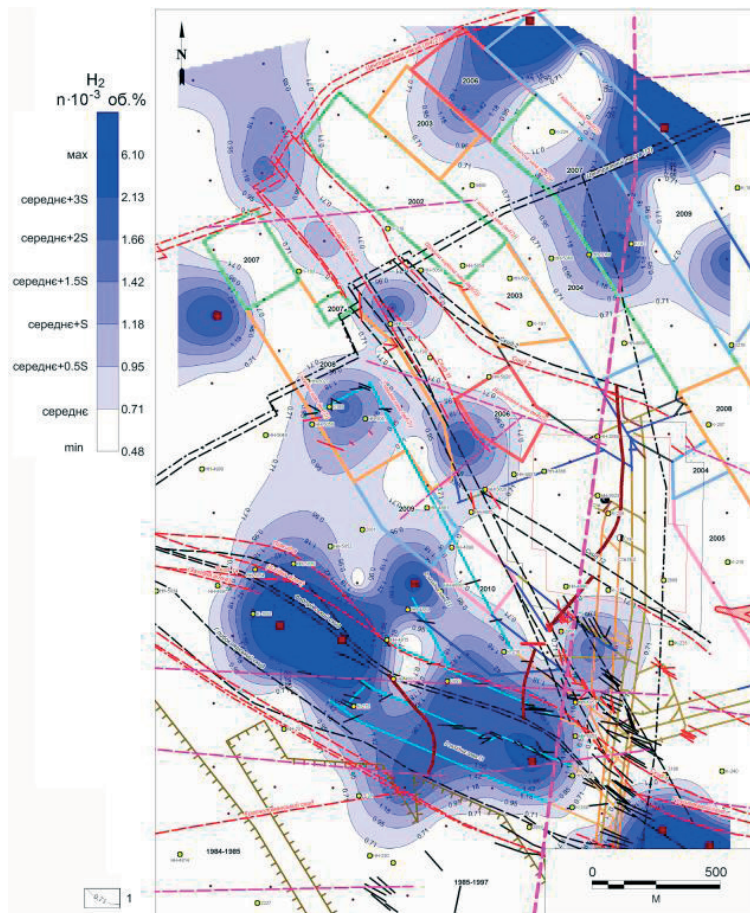
Рис. 12. Схема пространственного распределения показателей содержания водорода в подгрунтовой атмосфере на участке шахты «Краснолиманская»: 1 – изолинии показателей содержания водорода H_2 \cdot (n \cdot 10^{-3} \text{ об. } \%)
