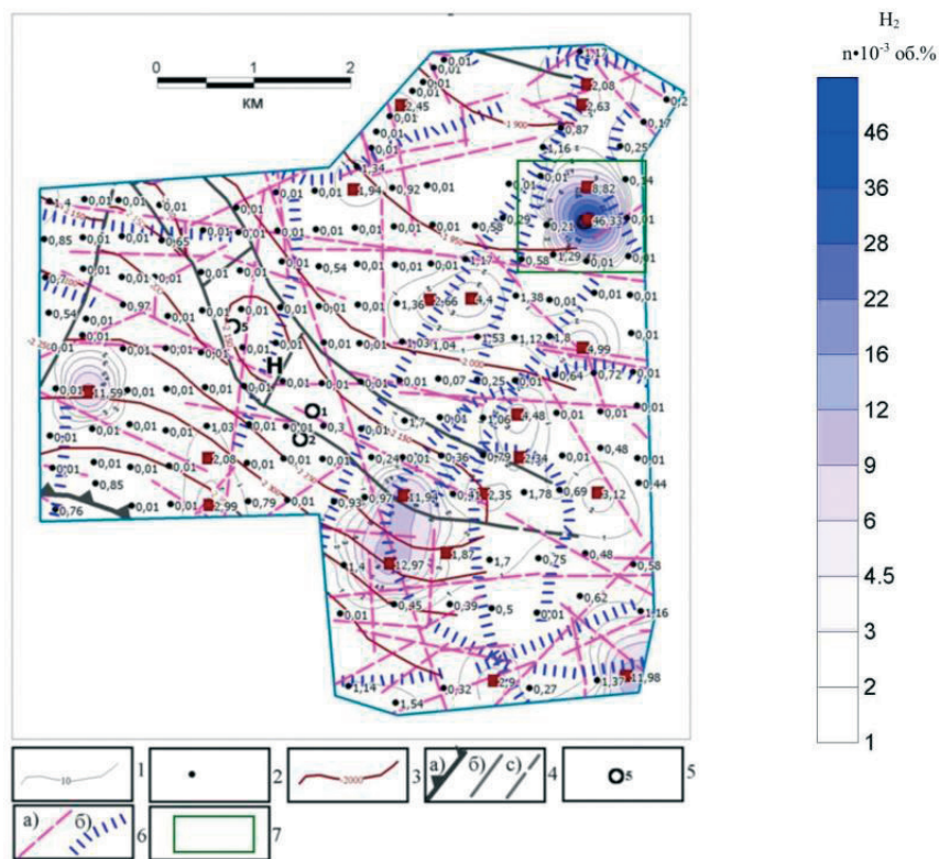
Рис. 4. Схема пространственного распределения показателей содержания водорода в подгрунтовом воздухе на Недельной площади (2006 г.):
