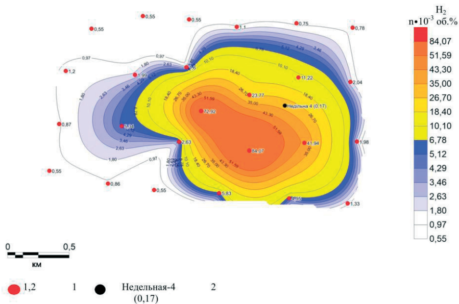
Рис. 6. Схема пространственного распределения показателей содержания водорода в подгрунтовом воздухе на детализационном участке Недельной площади: 1 – пункты наблюдений с измеренными значениями содержания водорода H_2 ( n \cdot 10^{-3} об. %); 2 – скв. Недельная-4 с измеренными значениями содержания водорода в скважине
