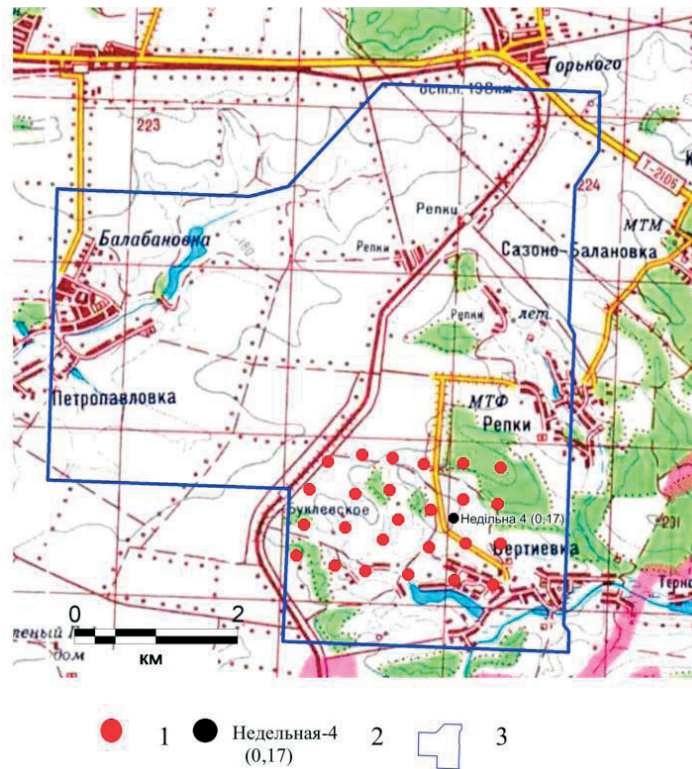
Рис. 5. Схема пространственного распределения пунктов наблюдений СТАГГИ на Недельной площади (на топографической основе м-ба 1 : 100 000): 1 – пункты наблюдений; 2 – скв. Недельная-4 с измеренными значениями водорода в скважине; 3 – контур исследований на Недельной площади
