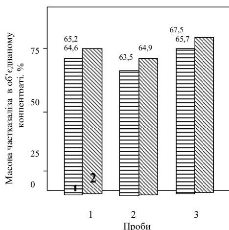
Рис. 1. Гістограми якісних показників магнітного аналізу проб пристайійній (1) і сумісній (2) стадій сепарації. Проби: 1 - гематит-магнетитова; 2 - магнетит - гематитова; 3 - гематит-силікат-магнетитова
