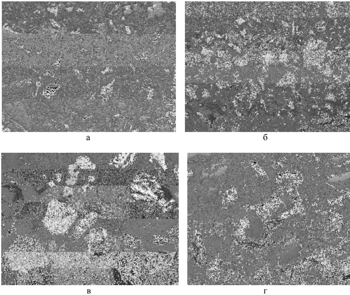
Рис. 1. Особенности минерального состава и строения частиц лежалых хвостов размером менее 0,1 мм (а, б) и более 0,1 мм (в, г).
