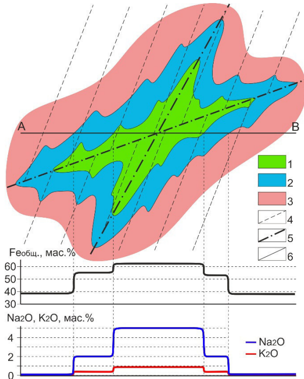
Рис. 3. Изменение (по разрезу АВ) содержания железа и оксидов щелочных металлов в схематическом разрезе зональной залежи руд первомайского вида.
