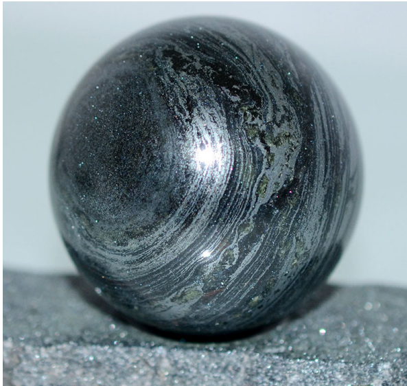
Рис. 1. Сувенірна куля, виготовлена із залізнослюдко-магнетитового кварциту Петрівського родовища зі згідним прожилком спекуляриту.
