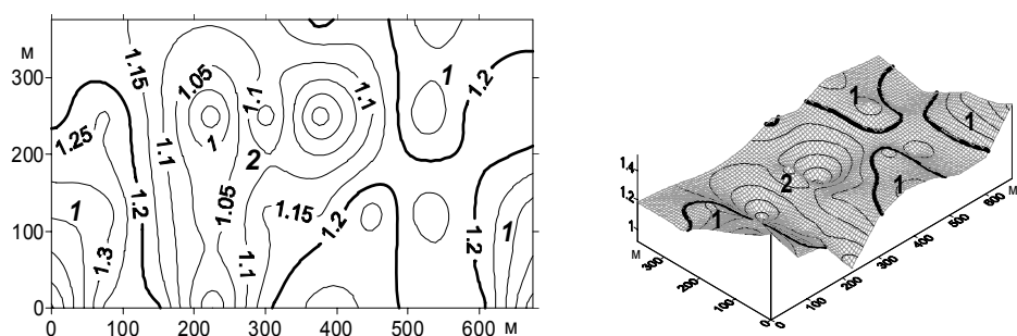
Рис. 6. Горизонтальный профиль почвенного покрова объекта Романив по неоднородности частного свойства (плотности сложения в посевном слое: 1 – >1,2 г/см 3 ; 2 – <1,2 г/см 3 )
