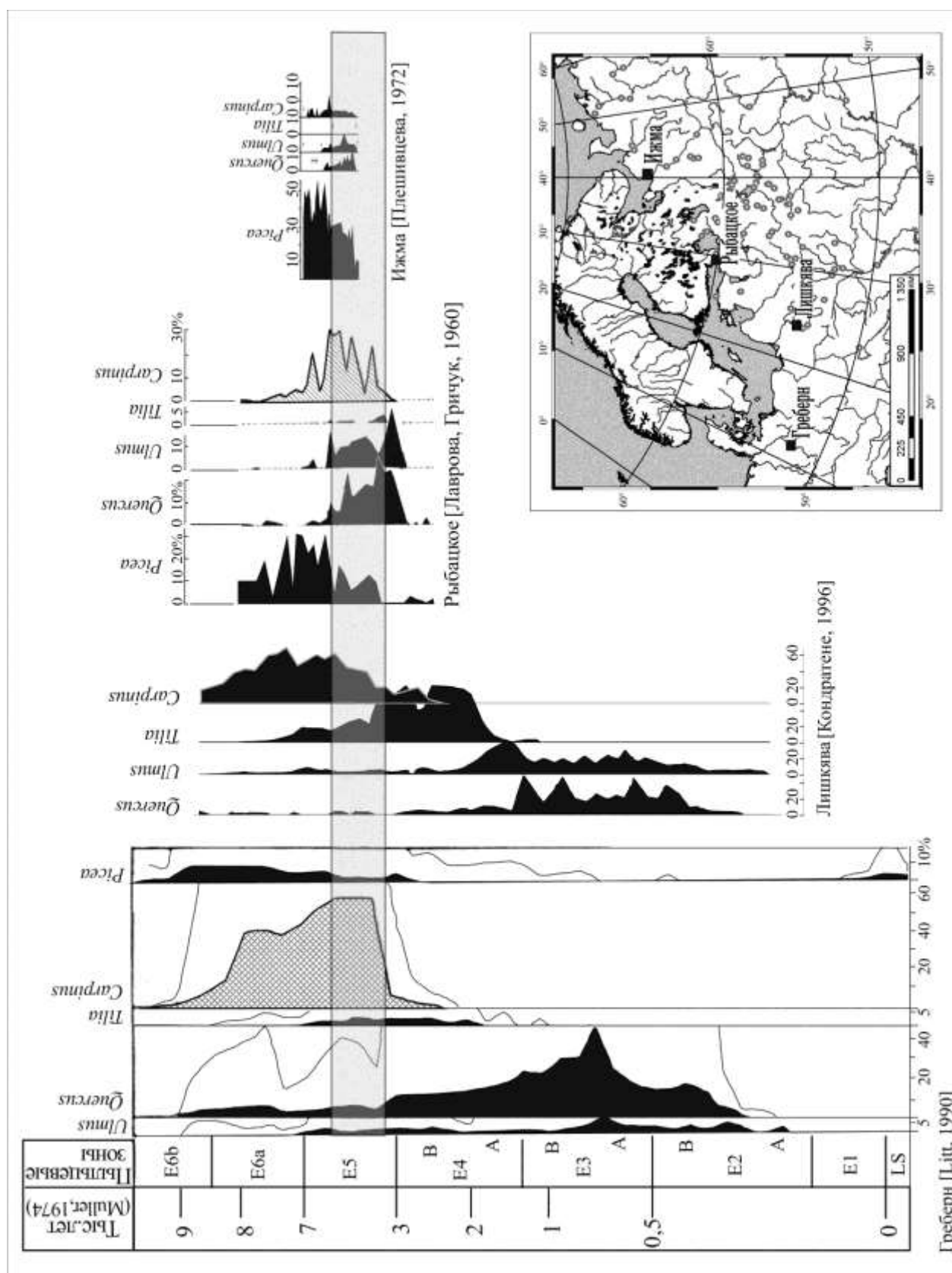
Рис.2. Хронологическая корреляция палинологических данных микулинского межледникова
