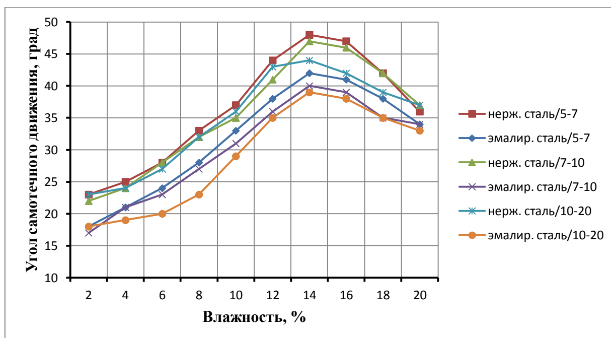
Рисунок 4 – График зависимости угла самотечного движения образцов от крупности породы ее влажности и типа используемой поверхности
