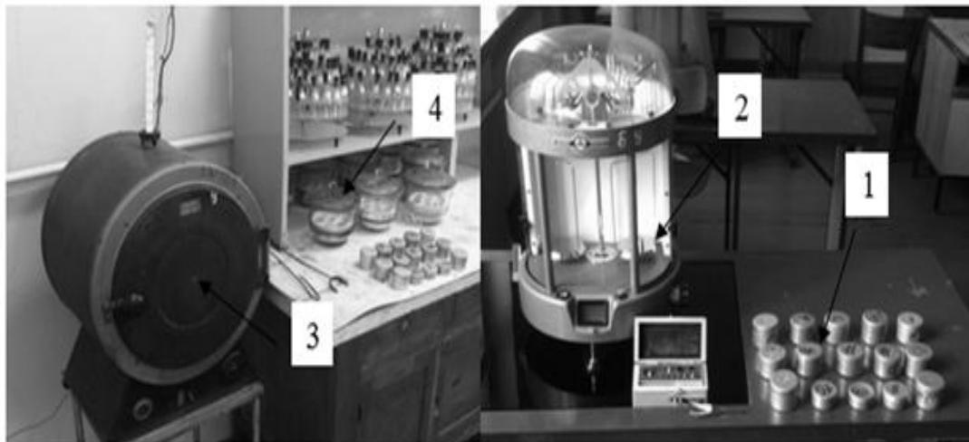
1- набор бьюксов; 2- аналитические весы; 3-сушильный шкаф; 4 эксикатор
