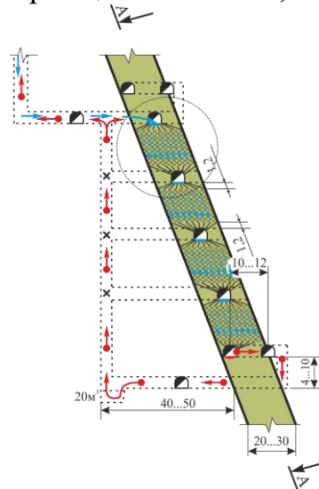
Рисунок 3 – Принципова схема видобутку урану методом хімічного вилуговування
