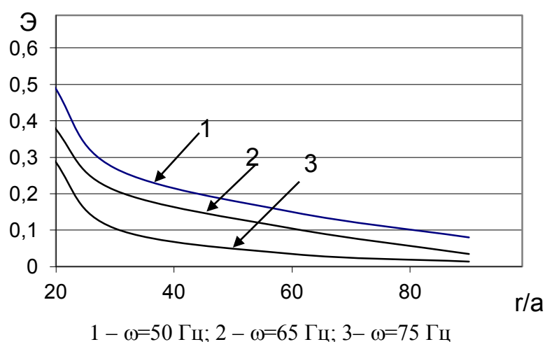
Рисунок 1 - Изменение параметра энергопередачи при вибровоздействии на смерзшуюся угольную среду при t = -10^\circ C с удалением от источника волнового возбуждения
