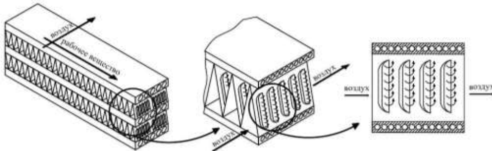
Рисунок 1 – Элемент теплообменной поверхности
