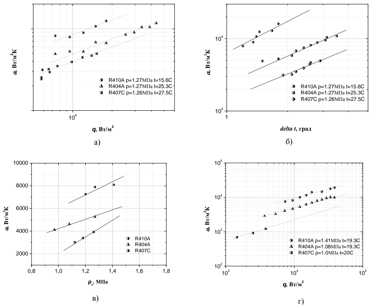
Рисунок 6 – Экспериментальные зависимости при развитии пузырькового кипения хладагентов R404a, R407c и R410a: а) \alpha=f(q) при давлении 1,26-1,27 МПа; б) \alpha=f(\Delta T) при давлении 1,26-1,27 МПа; в) \alpha=f(p_n) при q=9500 \text{ Вт/м}^2 ; г) \alpha=f(q) при температуре 19,3-20 °С
