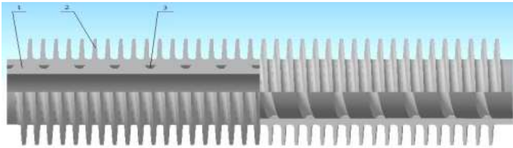
1 – внутренняя труба; 2 – наружная ребристая труба; 3 – БК Рисунок 4 – Биметаллическая ребристая труба с БК.
