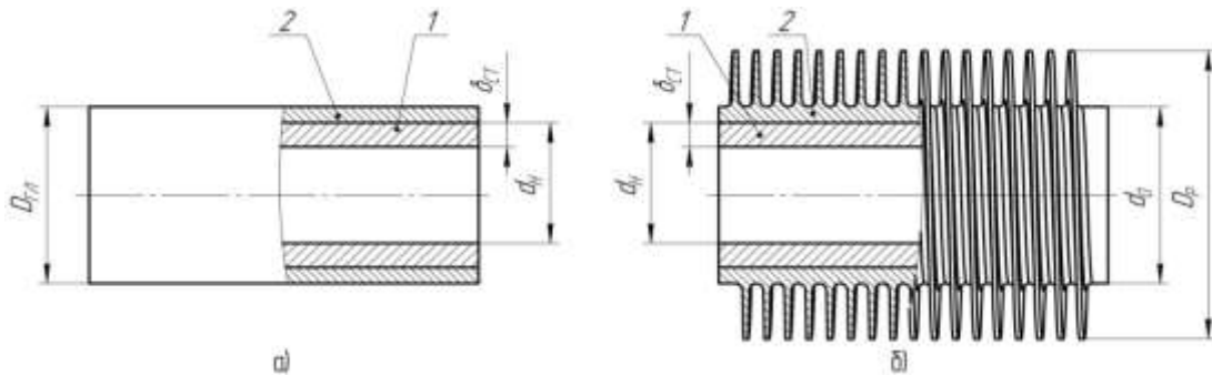
а) – биметаллическая гладкая труба; б) – биметаллическая ребристая труба; 1 – внутренняя труба; 2 – наружная гладкая/ребристая труба.
