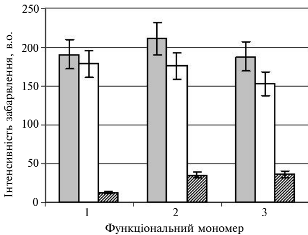
Рис. 1. Залежність інтенсивності забарвлення МІП (■) і контрольних (□) полімерних мембран, а також рівнів вибіркової адсорбції (▨) сульфаметоксазолу від типу функціонального мономера, застосованого при синтезі: 1 – МАК; 2 – ІК; 3 – АМПСК. Всі мембрани синтезовані з мономерних сумішей зі співвідношенням матриця:функціональний мономер = 1:2
