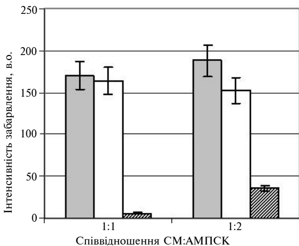
Рис. 2. Залежність інтенсивності забарвлення МІП (■) і контрольних (□) полімерних мембран, а також рівнів вибіркової адсорбції (▨) сульфаметоксазолу (СМ) від співвідношення матриця:функціональний мономер, застосованого при синтезі мембран. Функціональний мономер – АМПСК
