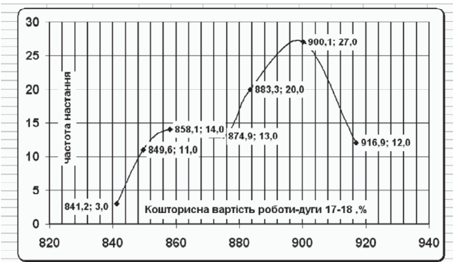
Рис. 3. Приклад проміжних результатів імітаційних блоків сіткової моделі: розподіл діапазону значень кошторисної вартості роботи-дуги №17-18 за частотами після 100 імітацій
