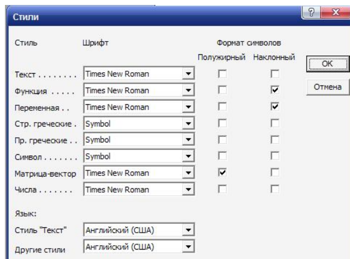
Рисунок 3 – Стиль формул
