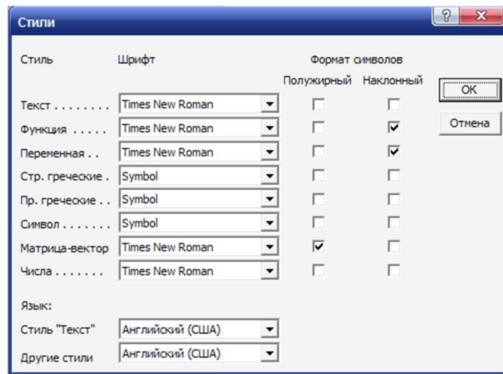
Рисунок 3 – Стиль формул
