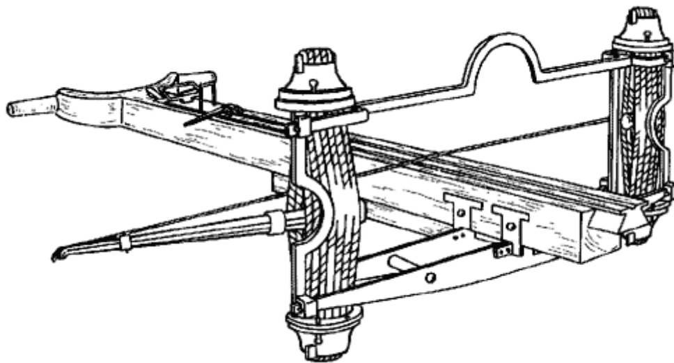
Рис. 18. Римська манубаліста (“ручна баліста”). Реконструкція Д. Баатца (D. Baatz). Джерело: http://xlegio.ru/throwing-machines/antiquity/handheld-ancient-artillery/ (25.07.2011)
