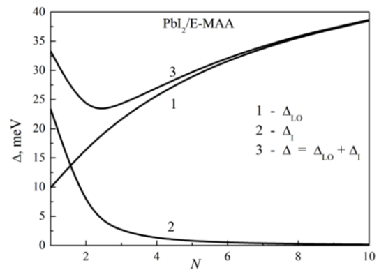
Рис. 2 – Залежність величини зміщення енергії дна найнижчої екситонної зони, зумовленого взаємодією з ЛО- та І-фононами від товщини НП
