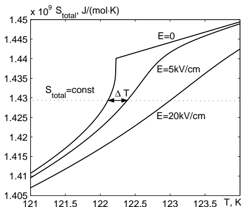
Рис. 1. Температурна залежність молярної ентропії кристалів \text{KH}_2\text{PO}_4 за різних величин поля.
