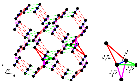
Рис. 1. Узагальнена ґратка голандиту (справа) утворена трикутними драбинками трьох типів. Її можна розбити на однакові тритрикутні кластери (зліва).
