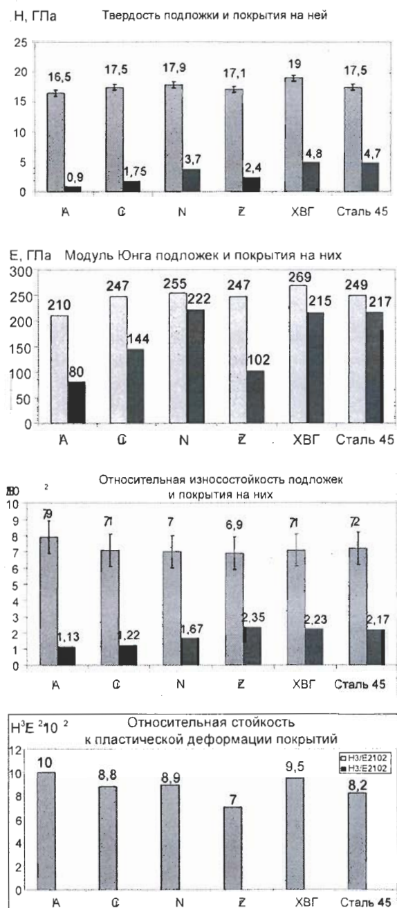
Рис. 5. Гистограммы механических свойств карбидохромовых покрытий и материалов подложек
