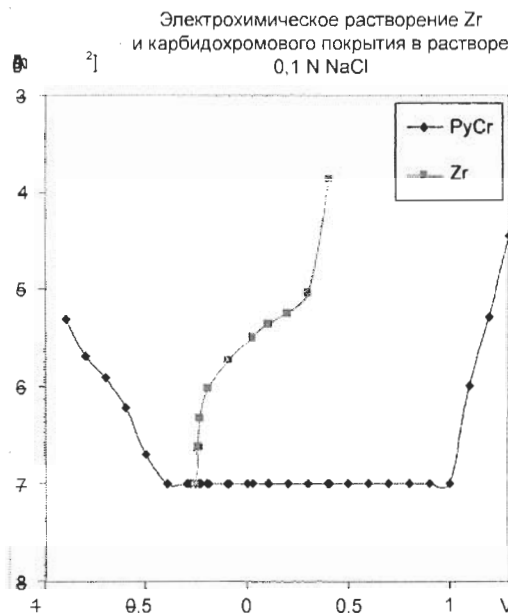
Рис. 7. Сравнительные электрохимические характеристики карбидохромового покрытия и Zr
