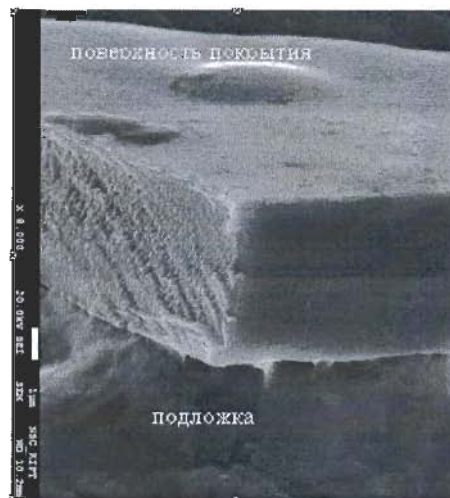
Рис. 13. Вид излома перпендикулярно поверхности роста карбидохромового покрытия
