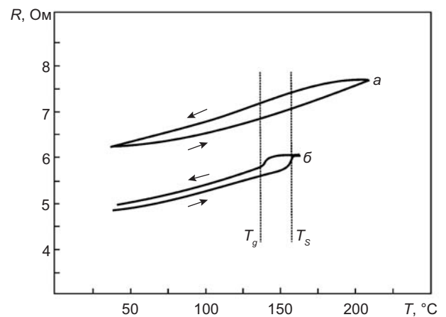
Рис. 5. Зависимость сопротивления в циклах нагрев-охлаждение от температуры для пленок Cu-In-Cu до ( а ) и после ( б ) нагрева до 350 °С
