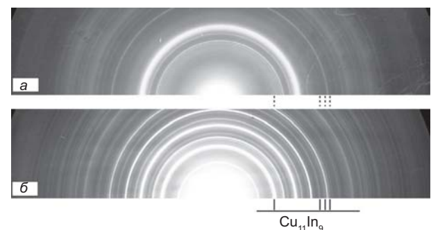
Рис. 6. Электронограммы пленок Cu-In до ( а ) и после ( б ) нагрева до 350 °С
