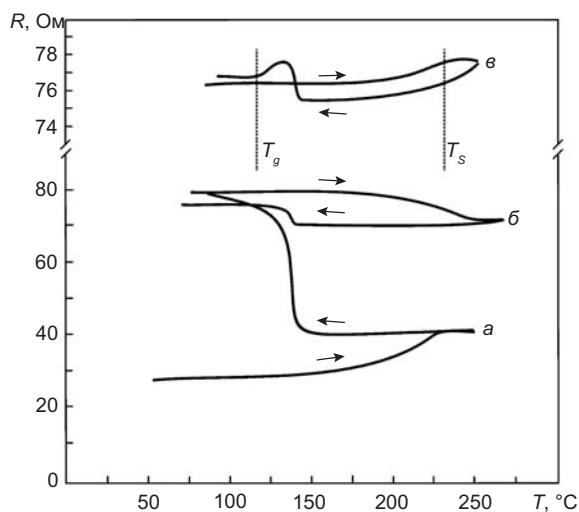
Рис. 4. Зависимость сопротивления от температуры для пленок Mo-Sn в первом ( a ), втором ( б ) и пятом ( в ) циклах нагрев-охлаждение
