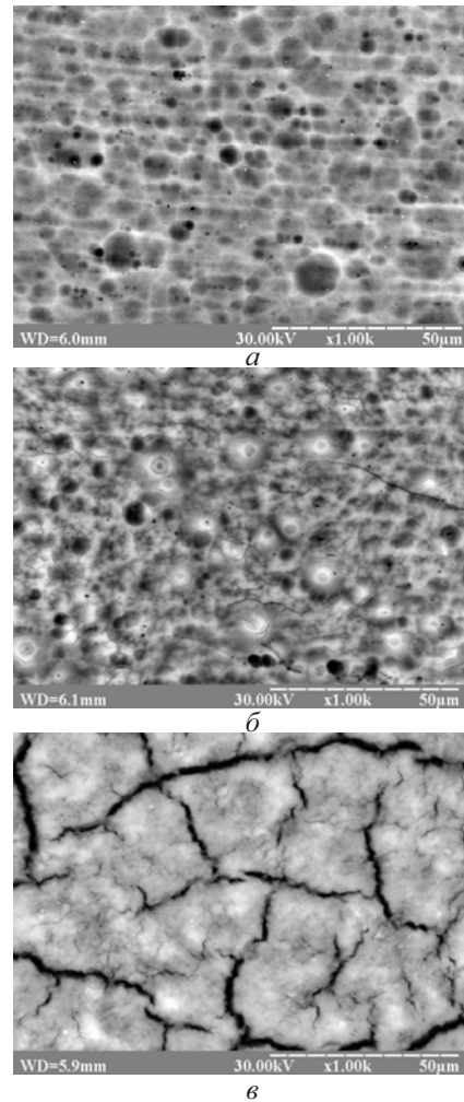
Рис. 2. Мікроскопічні знімки зразків серій № 2, № 4 та № 6 (а–в), отримані за допомогою растрового електронного мікроскопу РЕМ-106 при збільшенні у 1000 разів
