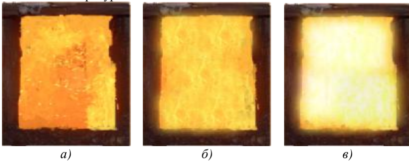
Рис. 2. Горіння мазутного палива в котлі ДКВР: а) - мазут М100; б) - 7% ВМЕ; в) - 15% ВМЕ.
