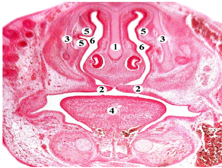
Рис. 4. Фронтальний зріз носової ділянки зародка щура 18,0 мм ТКД. Забарвлення гематоксилином і еозином. Мікропрепарат. Об. 4, ок. 7:
