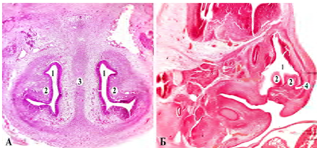
Рис. 3. Горизонтальний зріз голови зародка собаки 8,0 мм ТКД (А) та сагітальний зріз голови зародка щура 7,0 мм ТКД (Б). Забарвлення гематоксилином і еозином. Мікропрепарат. Об. 8, ок. 7:
