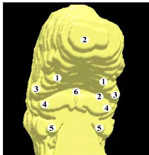
Рис. 2. Тривимірна комп'ютерна реконструкція верхньої половини зародка людини 7,0 мм ТКД. Передня права проекція. Зб. 1:60:
