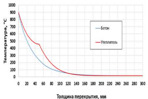
Рис. 7. Распределение температуры по высоте сечения плиты перекрытия через 60 мин при нагреве по режиму стандартного пожара.
