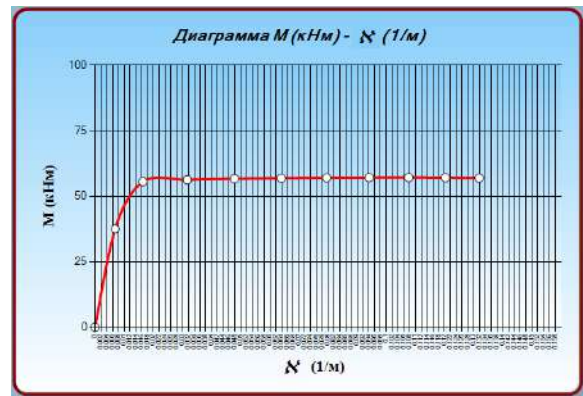
Рис. 9. Диаграмма изгибающий момент (кНм) – кривизна
