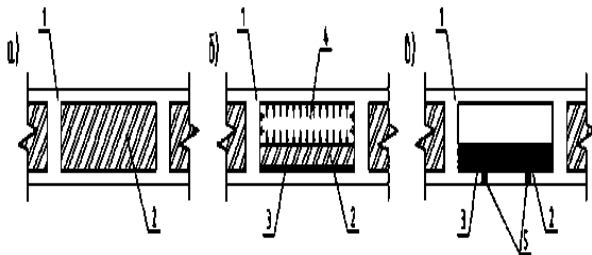
Рис. 2. Расчетные схемы, учитывающие флуктуации вкладыша-пустотообразователя
