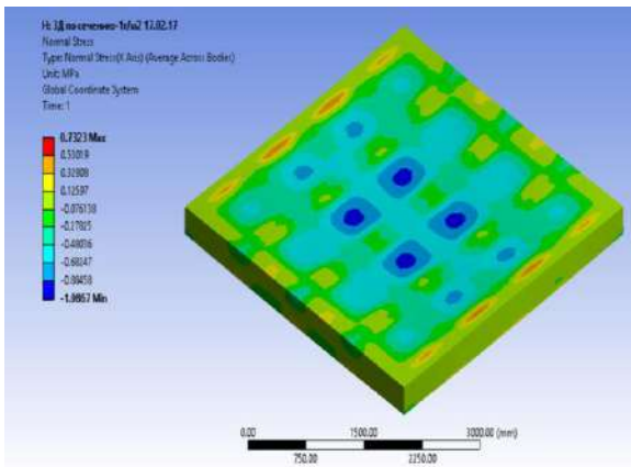
Рис.3.Результующиезначениянормальных напряжений пространственнойтрехмерноймоделиплиты.
