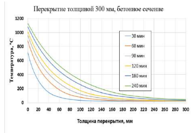
Рис. 5. Распределение температуры по высоте плиты перекрытия 300мм по бетонному сечению.
