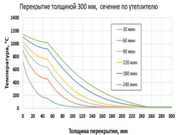
Рис. 6. Распределение температуры по высоте плиты перекрытия 300мм по утеплителю.
