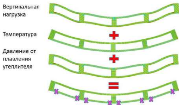
Рис. 8. Характер деформирования КЭ модели плиты перекрытия после 30 минут стандартного пожара.
