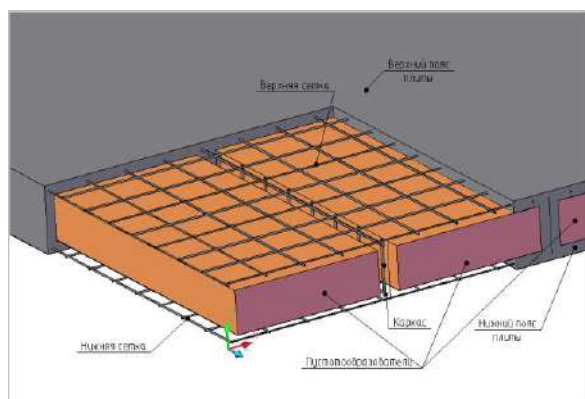
Рис. 1. Конструктивные особенности плиты конструктивной системы «Монофант».
