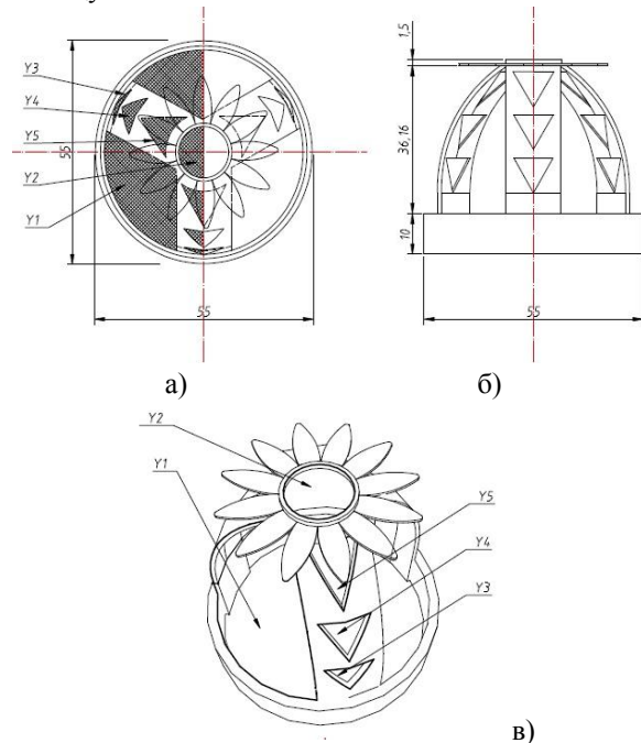
Рис. 2. Тепловий пожежний сповіщувач ИП-105 із ЗЗК «Мак1». а) Вид згори; б) Вид збоку; в) Інженерна візуалізація;
