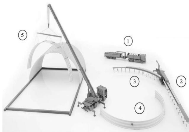
Рис. 2. Схема виробництва і монтажу збірних оболонкових систем
