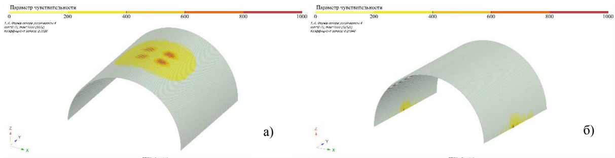
Рис. 22. Чутливість для 4-й форми втрати стійкості для: а) FEM-1; б) FEM-2
