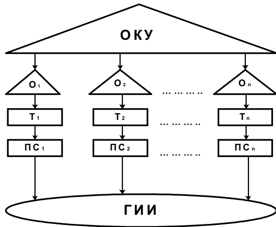
Рис. 3. Архитектура сети трансдисциплинарных знаний: O_1 - O_n – онтологии предметных областей; T_1 - T_n – формальное представление научных теорий; ПС_1 - ПС_n – соответствующие прикладные системы; ОКУ – онтология категориального уровня; ГИИ – глобальная информационная инфраструктура (next generation network).
