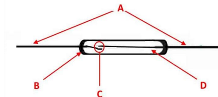
A — виводи геркона; B. — Скляна колба; C — контактна група; D — інертний газ або вакуум.
