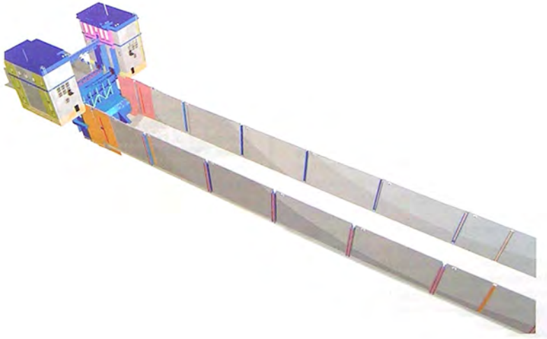
Рис. 13. Тривимірна метрична модель Новосибірського судноплавного шлюзу, точність якої складає 5-6 см
