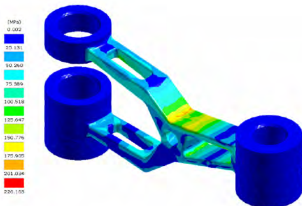
Рис. 14. Оцінювання коефіцієнта безпеки деталі
