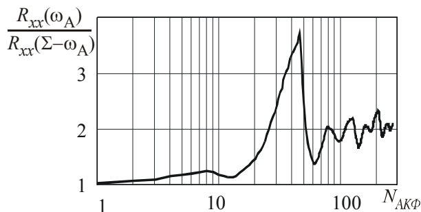
Рисунок 5 – Залежність відношення спектральної складової АКФ корисного сигналу до всіх інших складових спектру АКФ від N_{AK\Phi}
