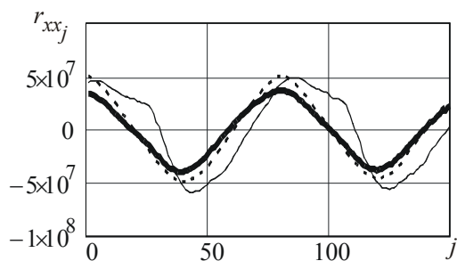
Рисунок 6 – АКФ вхідного сигналу при N_{AK\Phi} = 20 (суцільна тонка лінія), N_{AK\Phi} = 47 (штрихова лінія) і N_{AK\Phi} = 80 (суцільна товста лінія)
