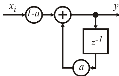
Рисунок 3– Структура авторегресійного фільтра першого порядку
