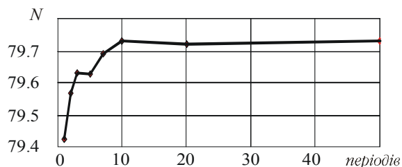
Рисунок 9 – Залежність кількості відліків на період досліджуваного сигналу від кількості усереднених періодів
