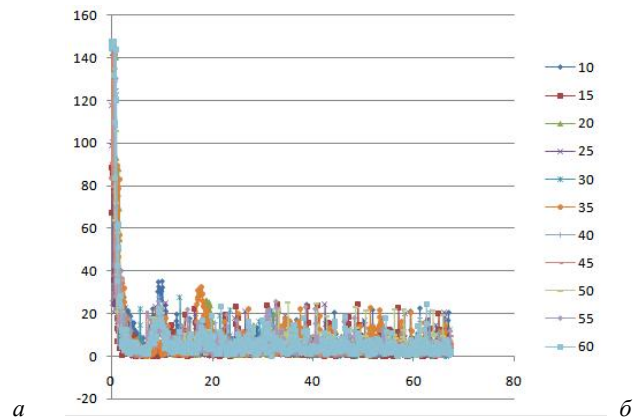
Рис. 5. Вимірювальний діапазон за температури 10 °С (а); сигнал за різних температур від 10 до 60 °С (б) Fig. 5. Image of measuring at the temperature of 10 °C (a); signal at different temperatures from 10 to 60 °C (b)
