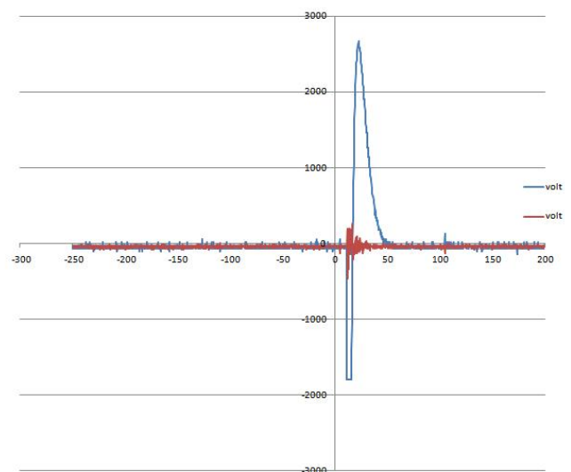
Рис. 7. Отриманий сигнал за температури 60 °С Fig. 7. Got signals at a temperature 60 °C
