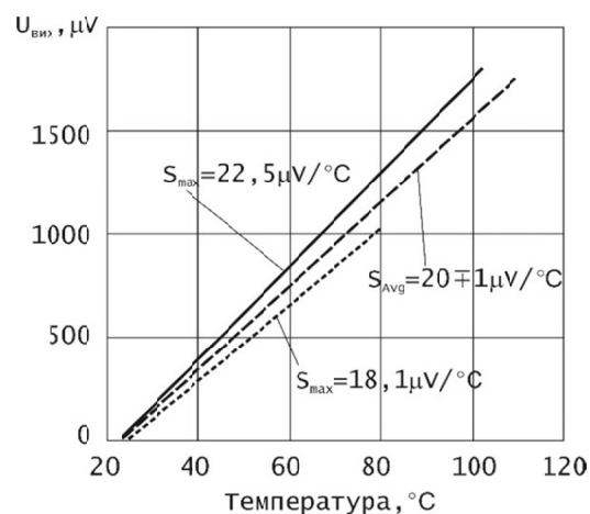
Рис. 6. Градувальні залежності для групи із 20 термоперетворювачів [6]
