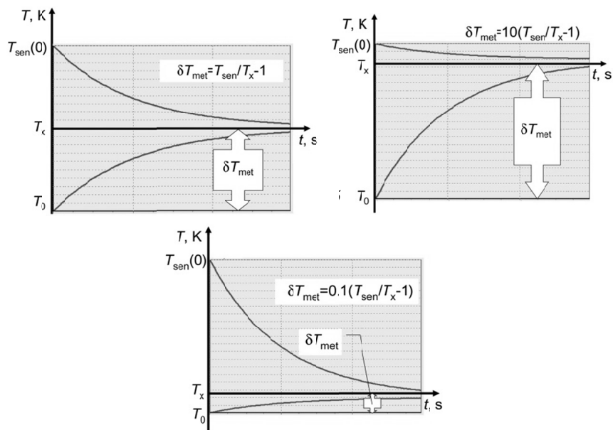
Рис. 1. Часові зміни температури за контакту «теплого» сенсора вихідної температури T_{sen}(0) з «холодним» об'єктом вихідної температури T_0 : a - c_{ob}w_{ob}V_{ob} = c_{sen}w_{sen}V_{sen} ; b - 10c_{ob}w_{ob}V_{ob} = c_{sen}w_{sen}V_{sen} ; c - c_{ob}w_{ob}V_{ob} = 10c_{sen}w_{sen}V_{sen} .
