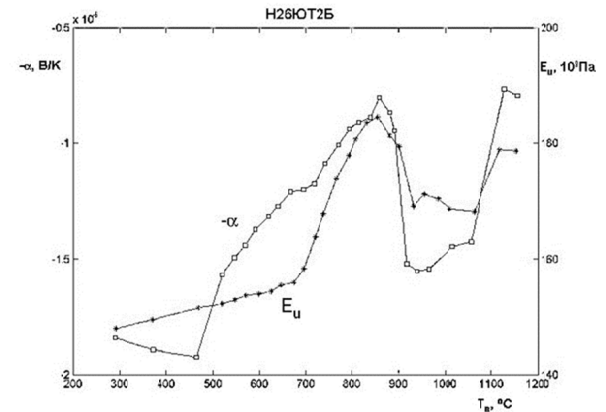
Рис. 4. Залежність абсолютної термо-ЕРС \alpha та модуля Юнга E_u сплавів H26ЮТ3 (а), H26ЮТ2Б (б) від температури відпуску T_B
