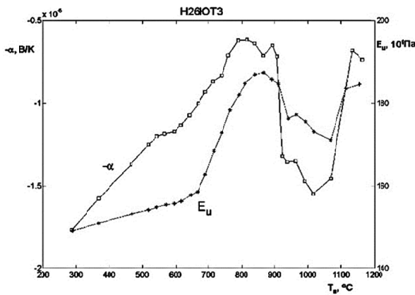
Рис. 4. Залежність абсолютної термо-ЕРС \alpha та модуля Юнга E_u сплавів H26ЮТ3 (а), H26ЮТ2Б (б) від температури відпуску T_B
