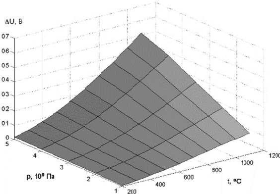
Рис. 3. Ізобаричні поправки \Delta U для показів платинородій-платиногого термоперетворювача ПР 10/0
