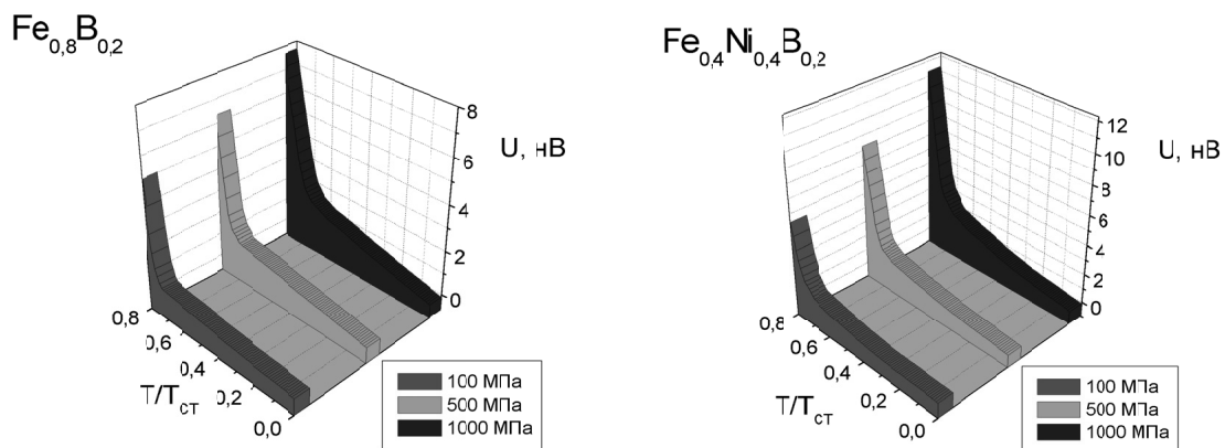
Рис. 7. Температурна залежність (T/T_{ст}) змін інтегральної термо-ЕРС U металевого скла для різних зусиль розтягування (100, 500 та 1000 МПа)
