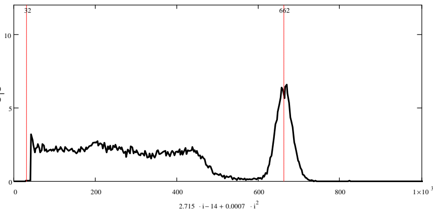
Рис. 5. Апаратурний відгук спектра для гамма-детектора CsI від ДІВ 137 Cs у тонкій капсулі зі сталі на установці УПД-2
