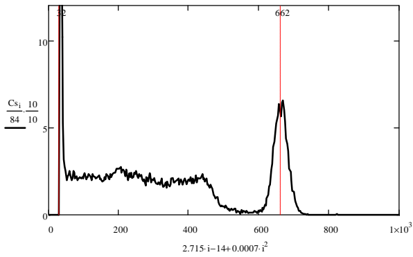
Рис. 2. Апаратурний відгук спектра від точкового джерела 137 Cs для гамма-детектора CsI
