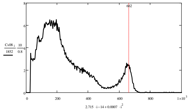
Рис. 3. Апаратурний відгук спектра для гамма-детектора CsI від ДІВ 137 Cs на установці УПД-Інтер з декількома атенюаторами із вольфрамового сплаву
