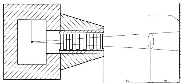
Рис. 1. Приклад колімованої установки
