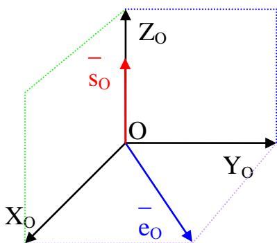
Рис. 3. Вектор \bar{S}_o расположен вдоль оси OZ_o ; вектор \bar{E}_o расположен в плоскости X_o Y_o
