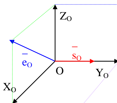
Рис. 4. Вектор \bar{S}_o расположен вдоль оси OY_o ; вектор \bar{E}_o расположен в плоскости Z_o X_o
