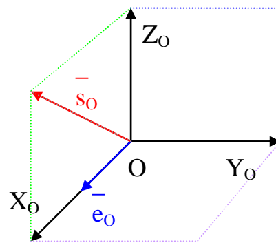
Рис. 6. Вектор \bar{E}_o расположен вдоль оси OX_o , а вектор \bar{S}_o расположен в плоскости Z_oX_o
