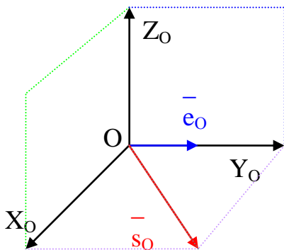
Рис. 5. Вектор \bar{E}_o расположен вдоль оси OY_o , а вектор \bar{S}_o расположен в плоскости X_oY_o
