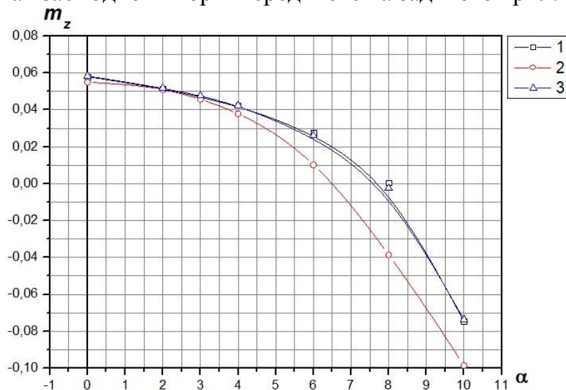
Рис. 7. Залежність коефіцієнта моменту тангажа від кута атаки: 1. моделі без вінглетів; 2. моделі із вінглетами на передньому крилі; 3. моделі із вінглетами на обох крилах
