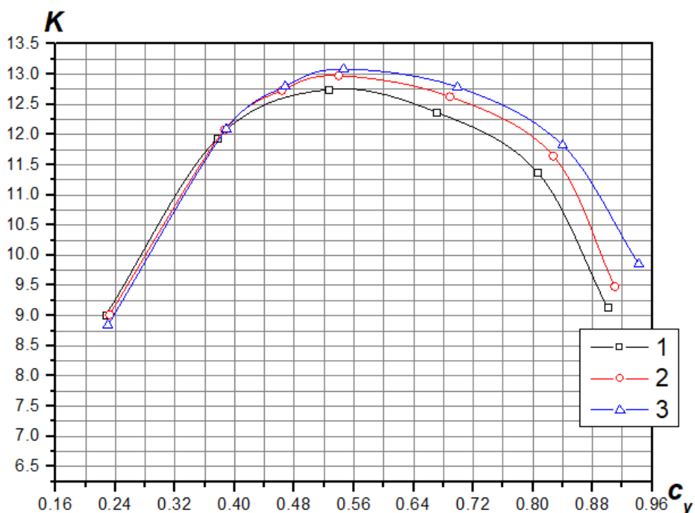
Рис. 6. Залежність аеродинамічної якості від коефіцієнта підйімальної сили для розрахункової сітки більшої розмірності: 1. модель без вінглетів; 2. модель із вінглетами на передньому крилі; 3. модель із вінглетами на обох крилах
