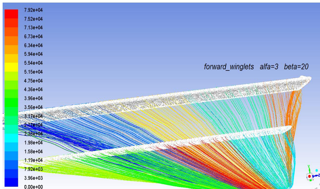
Рис. 10. Лінії току для системи двох крил із вінглетами на передньому крилі.
