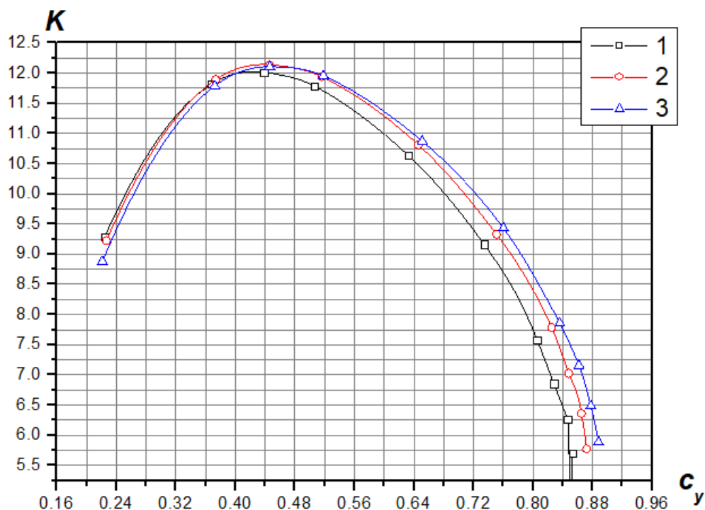
Рис. 5. Залежність аеродинамічної якості від коефіцієнта підйімальної сили: 1. без вінглетів; 2. із вінглетами на передньому крилі; 3. із вінглетами на обох крилах
