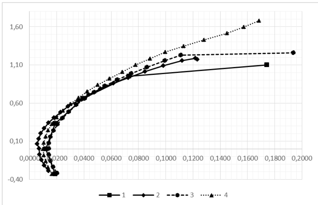
Рис. 3. Залежність коефіцієнта підйомної сили від коефіцієнта опору: 1 – експериментальні дані; 2 – модель із «приєднаним» крилом; 3 – моделі з «неприєднаним» крилом; 4 – масштабована модель
