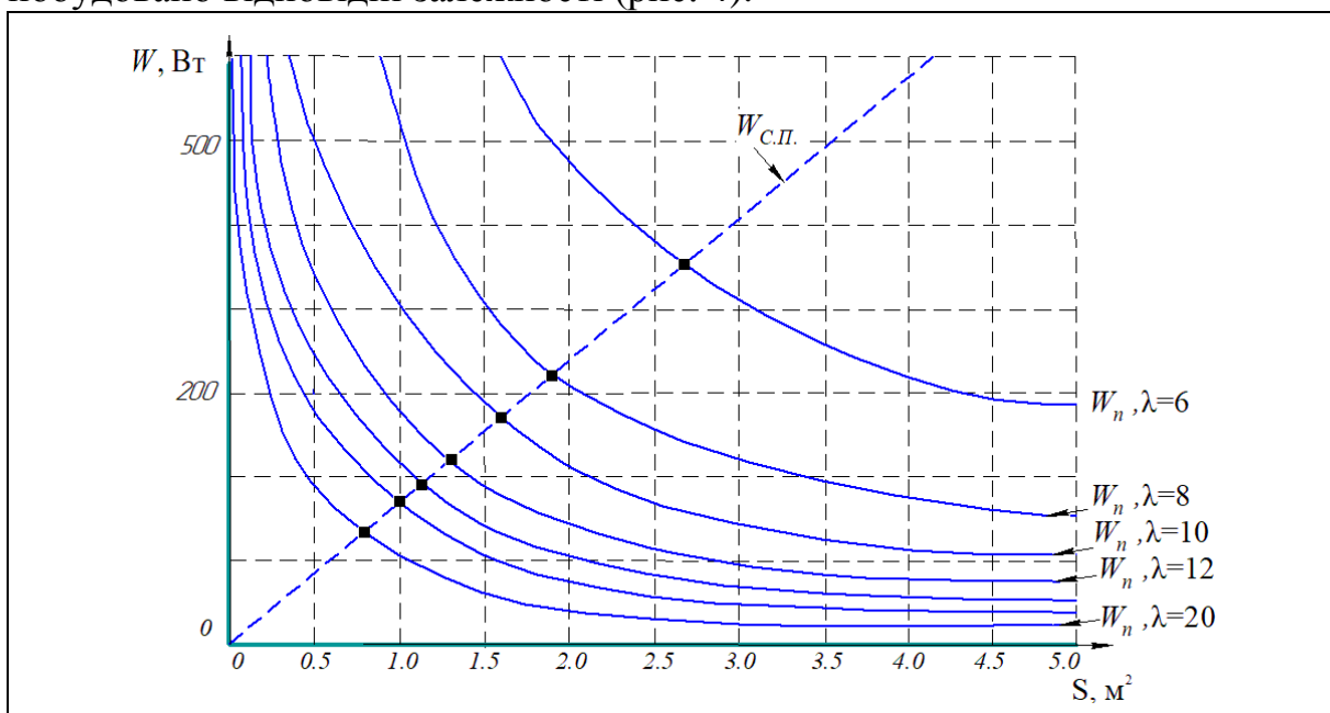
Рис. 4. Залежність потрібної W та наявної потужності W_n від площі крила S для різних його конфігурацій (різних видовженнях \lambda )
