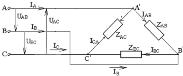
Рис.1. Трёхфазная электрическая цепь
