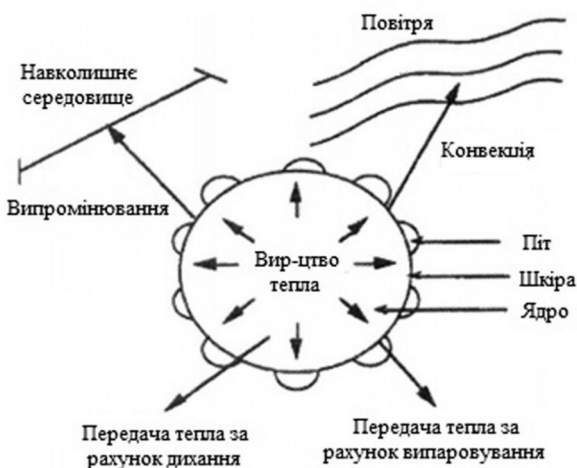
Рис. 1. Схематичний вигляд моделі Гадже [4]
