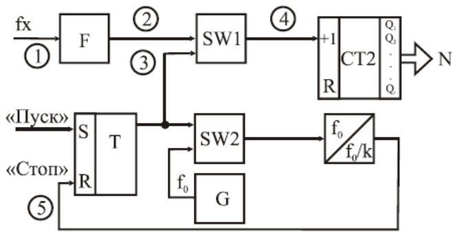
Рис. 2. Цифровий частотомір: Т-RS — тригер, SW2 — схема збігу, G — генератор зразкової частоти, ПЧ — подільник частоти, що формує зразковий часовий інтервал t_0
