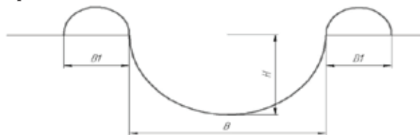
Рис. 1. Схема создания минерализованной полосы плугами
