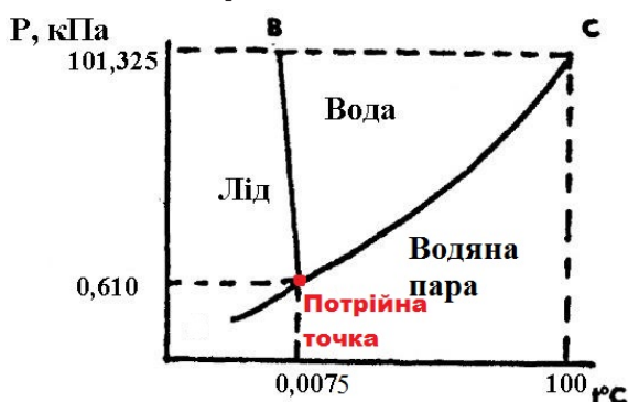
Рис. 1. Діаграма рівноваги фаз
