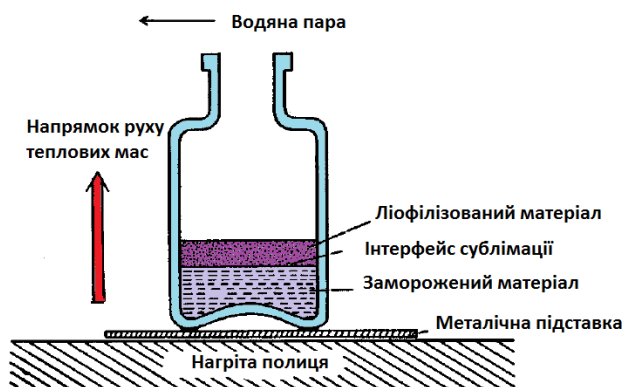
Рис. 2. Просторова модель флакона з матеріалом, що ліофілізується
