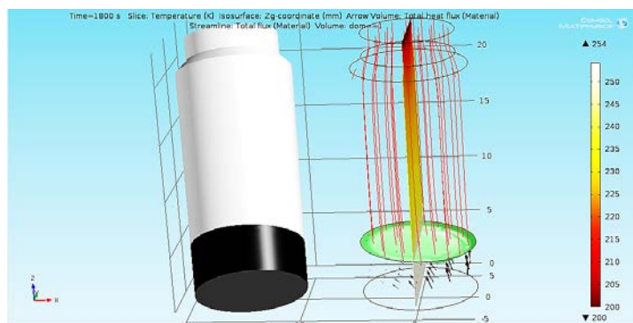
Рис. 4. 3D-модель процесу ліофілізації
