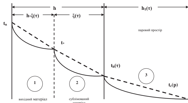
Рис. 3. Плоский переріз матеріалу та газового простору
